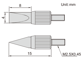
6282-1001
