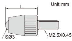
6282-0101
