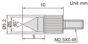
6282-0601
